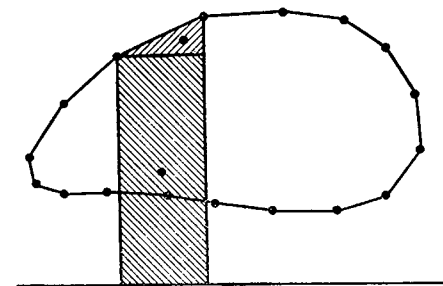
Рис. 5.36. Определение центроида трапециевидной аппроксимации.
