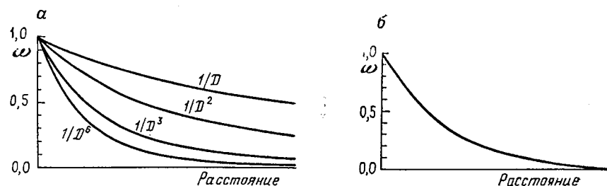
Рис. 5.56. Примеры взвешивающих функций от расстояния, используемых в программах построения карт в изолиниях:
