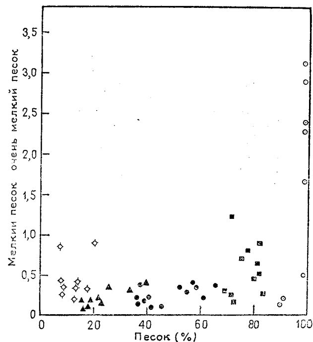
Рис. 6.32. Диаграмма зависимости содержания песка от отношения содержания тонкозернистого песка к очень тонкозернистому в осадках залива Баратария. Символы те же, что и на рис. 6.30
