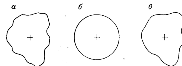
Рис. 5.39. Сравнение оцифрованного контура песчинки ( a ) с нулевой гармоникой или окружностью среднего радиуса ( б ) и с контуром, построенным по шести гармоникам ( в )
