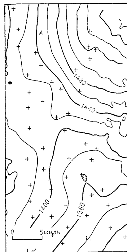
Рис. 5.67. Карта уровней воды в Экус Бедз, большом водоносном слое в южной части Центрального Канзаса.
