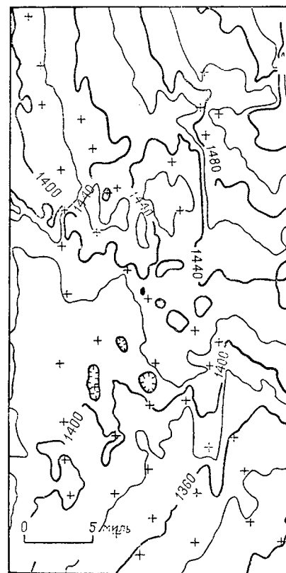
Рис. 5.69. Карта, представляющая дрифт первого порядка уровней воды в Экус Бедз.
