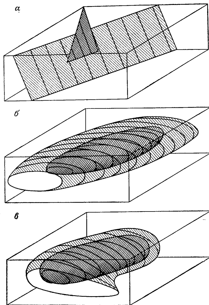
Рис. 5.88. Четырехмерные полиномиальные поверхности тренда для содержаний урана.
