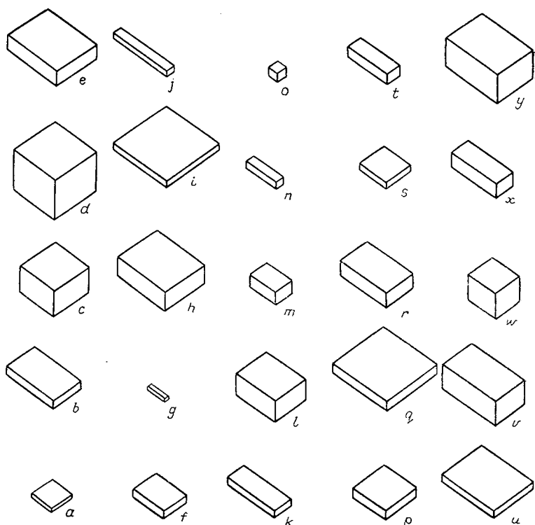
Рис. 6.16. Двадцать пять блоков со случайными значениями длины, ширины и высоты.
