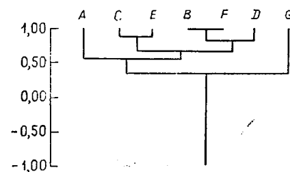
Рис. 6.10. Дендрограмма корреляционной матрицы, приведенной в табл. 6.15. Группы построены по методу прямой связи. Коэффициент корреляции равен 0,71
