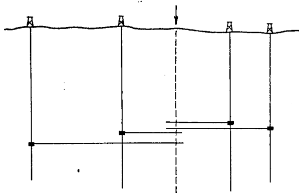
Рис. 5.52. Вид разреза, на котором представлены контрольные точки (скважины) с известными отметками поверхности (кровли формации). Оценки в узле сети (стрелка) сделаны в результате горизонтального проектирования и последующего усреднения
