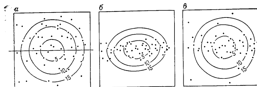
Рис. 5.86. Влияние распределения контрольных точек на поверхность тренда: a — исходная поверхность со случайным расположением контрольных точек; b — возмущенный тренд, полученный путем опробования исходной изучаемой поверхности в узкой полоске; v — почти правильный тренд, полученный путем добавления нескольких дополнительных точек за пределами узкой полосы наблюдений
