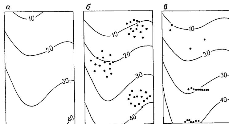
Рис. 5.87. Влияние группировки контрольных точек на поверхности тренда: a — исходная поверхность тренда третьей степени; б — поверхность тренда, полученная по контрольным точкам, расположенным группами; в — поверхность тренда, полученная по контрольным точкам, расположенным по частичным пересечениям проверяемой поверхности
