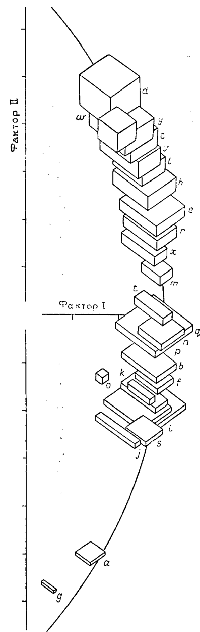
Рис. 6.39. Графическое представление факторных нагрузок Q-метода на первые две факторные оси для данных по блокам, вычисленных по матрице сходства \cos \theta (см. табл. 6.28).
