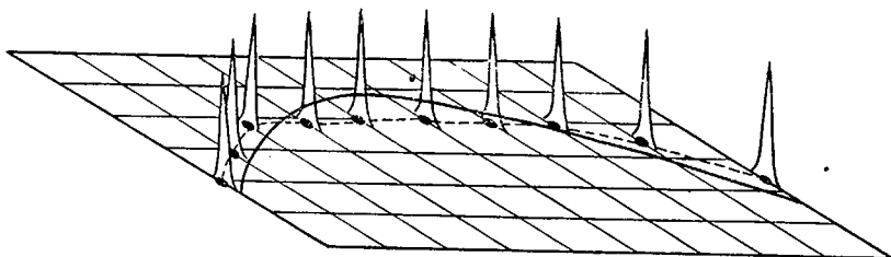
Рис. 5.85. Распределение случайной компоненты относительно наблюдаемой поверхности, соответствующей структурной модели поверхности тренда.
