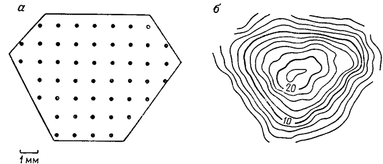
Рис. 5.83. (а) Расположение точек анализа в кристалле сфалерита (анализ выполнен под электронным микроскопом); (б) изолинии, характеризующие содержание железа
