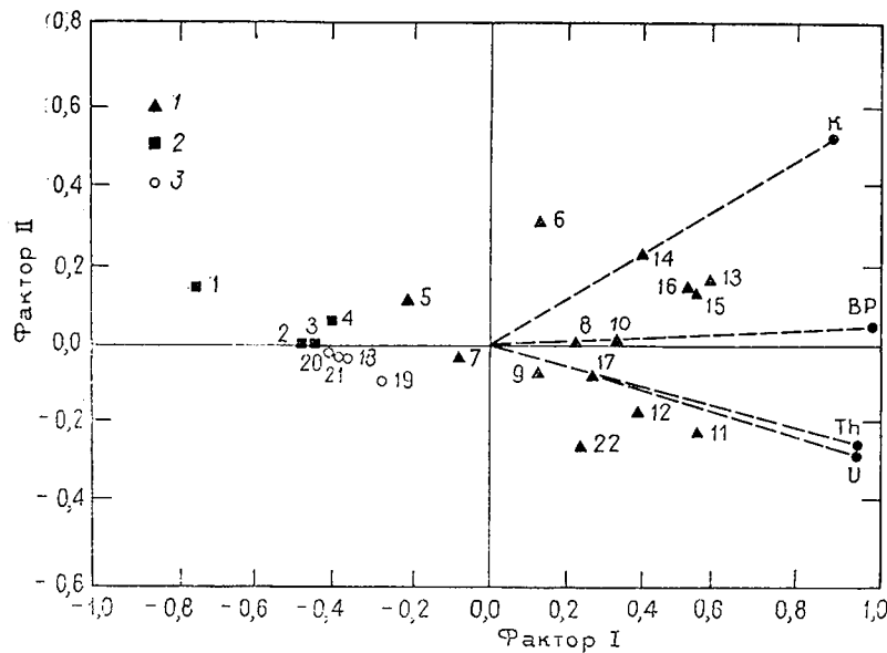
Рис. 6.50. Представление нагрузок R- и Q-методов на две первые факторные оси для данных Береа, вычисленных из ковариационной матрицы (см. табл. 6.42) [65].
