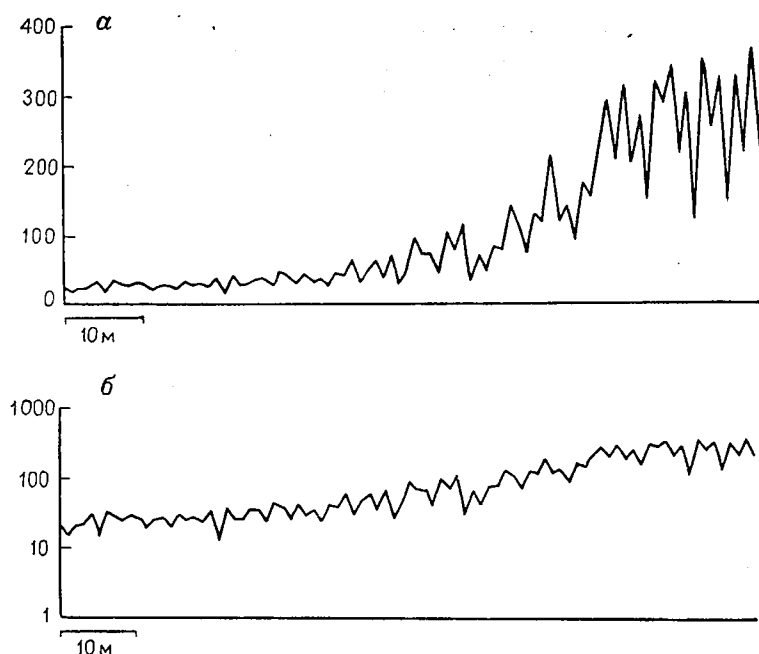
Рис. 5.60. Изменчивость содержаний серебра вдоль штольни рудника в Мексике:
