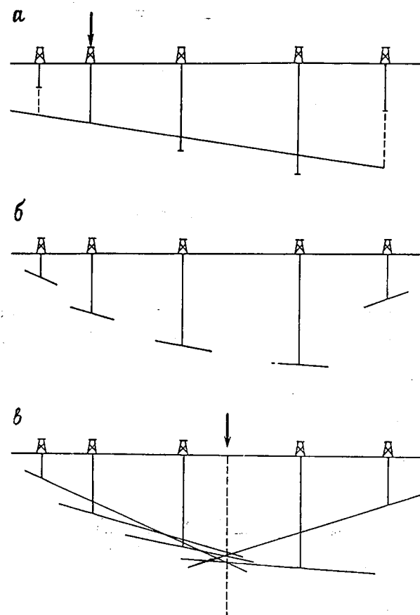
Рис. 5.55. Интерполяция для равномерно расположенных точек сети с помощью метода проектирования падения, который требует вычисления локального падения в каждой данной точке (изображено в разрезе) [69]:
