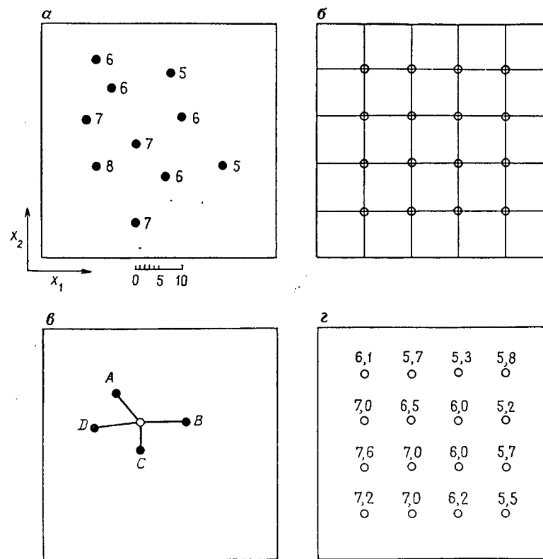
Рис. 5.53. Последовательность вычислений для построения изолиний при нахождении значений в узлах сети:
