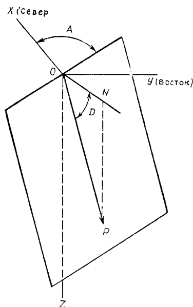
Рис. 5.28. Обозначения для трехмерного вектора, характеризующего простираение и падение.
