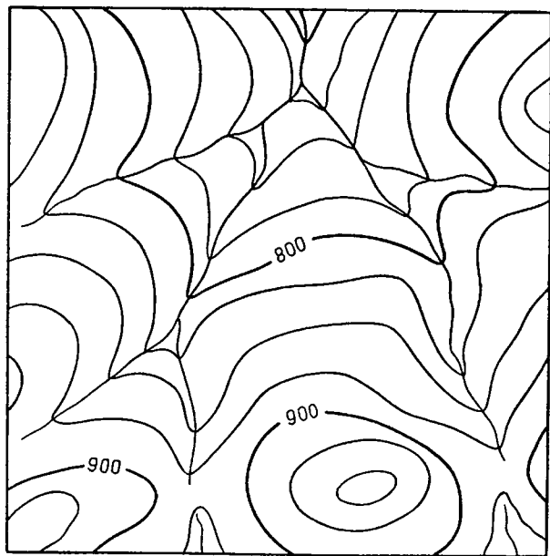
Рис. 5.59. Карта в изолиниях, построенная по топографическим данным вручную.
