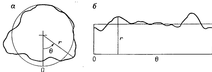
Рис. 5.37. Эквивалентность между полярными и декартовыми представлениями координат:
