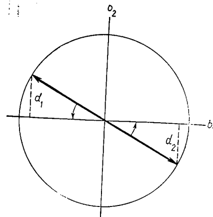
Рис. 5.30. Проекция двух диаметрально противоположных векторов на собственный вектор b_1 . Расстояния d_1 и d_2 идентичны и имеют одинаковый вращательный момент
