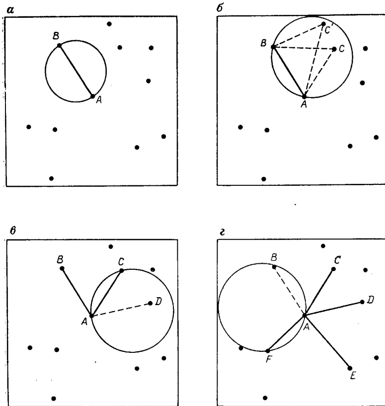
Рис. 5.47. Определение Тиссеновских соседей точки А:
