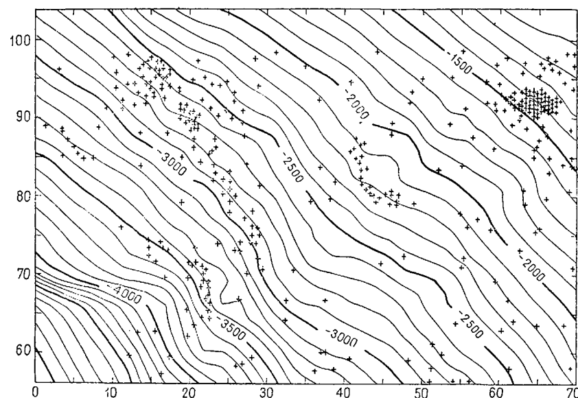
Рис. 5.76. Структурная карта вершины скал Бейзил-Фиш, бассейн Альберта. Изолинии указаны в футах ниже уровня моря. Крестики — контрольные скважины
