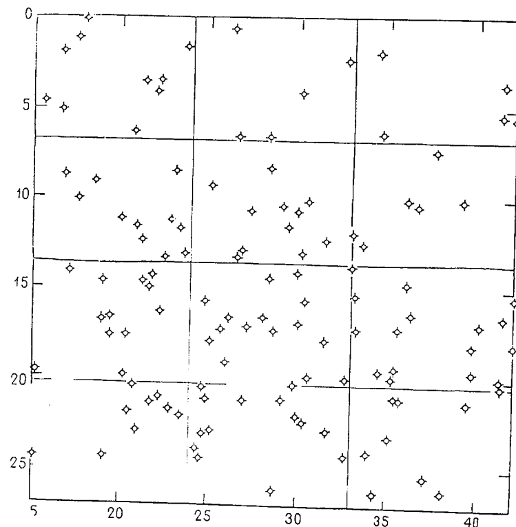
Рис. 5.10. Расположение 123 скважин, пробуренных в верхних слоях ордовикских отложений в Центральном Канзасе. Карта разделена на 12 ячеек одинакового размера
