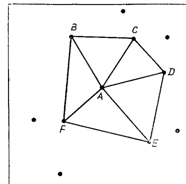
Рис. 5.48. Соединяя Тиссеновских соседей точки А, получаем треугольную сеть вокруг точки А. Процесс затем повторяют для одной из точек В—F и затем опять повторяют
