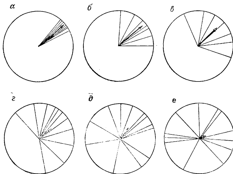
Рис. 5.22. Множества единичных векторов, иллюстрирующие значение, получаемое при различном расположении векторов во всех примерах, среднее направление — 52^\circ :
