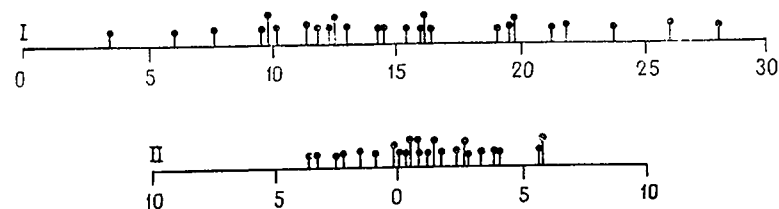
Рис. 6.21. Проекция точечных данных табл. 6.19 на главные компоненты. Дисперсия по компоненте I равна 37,9, а дисперсия по компоненте II — 6,5
