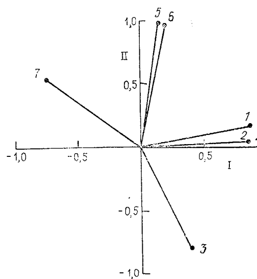
Рис. 6.37. Графическое представление тех же нагрузок после вращения по методу варимакс.
