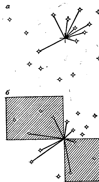
Рис. 5.57. (а) Метод поиска, локализуя n ближайших соседей вокруг оцениваемого узла сети. На радиальное распределение контрольных точек не накладывается никаких ограничений. (б) Схема поиска по квадратам, используемая для установления истинного распределения контрольных точек вокруг оцениваемых узлов сети. (в) Октантный вариант схемы поиска вокруг оцениваемых узлов сети
