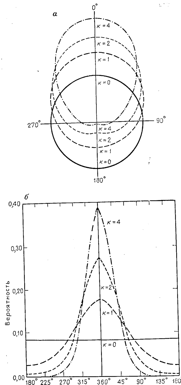
Рис. 5.24. Распределения фон Мизеса, имеющие различные параметры концентрации [33]:
