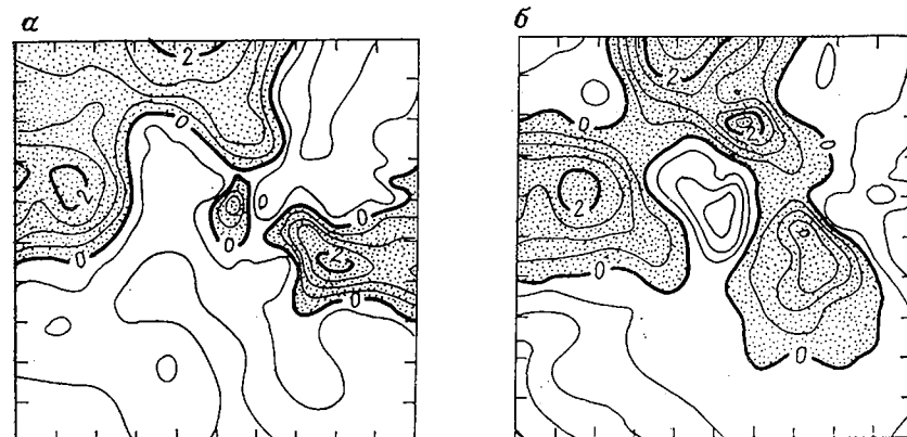
Рис. 5.103. Изменчивость стандартизованных параметров размера частиц донных осадков, собранных на побережье Северной Каролины (карты исходных параметров представлены на рис. 5.97):
