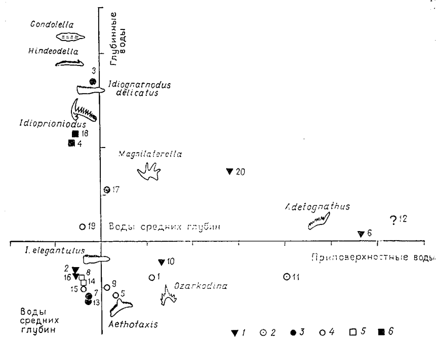
Рис. 6.44. Представление факторных нагрузок метода соответствия для данных по распространности конodontов, представленных в табл. 6.37.
