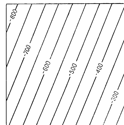
Рис. 5.74 Карта поверхности тренда по скважинам рис. 5.73.
