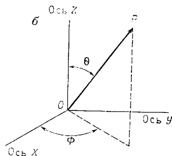
Рис. 5.27. Система обозначений векторов в трехмерном пространстве:
