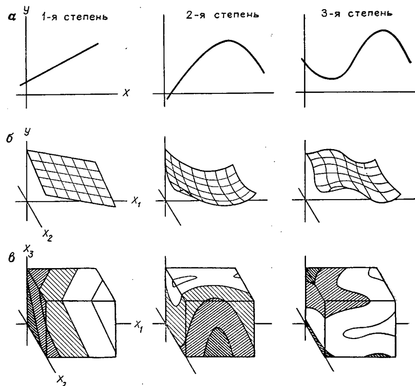
Рис. 5.90. Тренды от одной (а), двух (б) и трех (в) независимых переменных, полученные по полиномиальным уравнениям первой, второй и третьей степеней [37]
