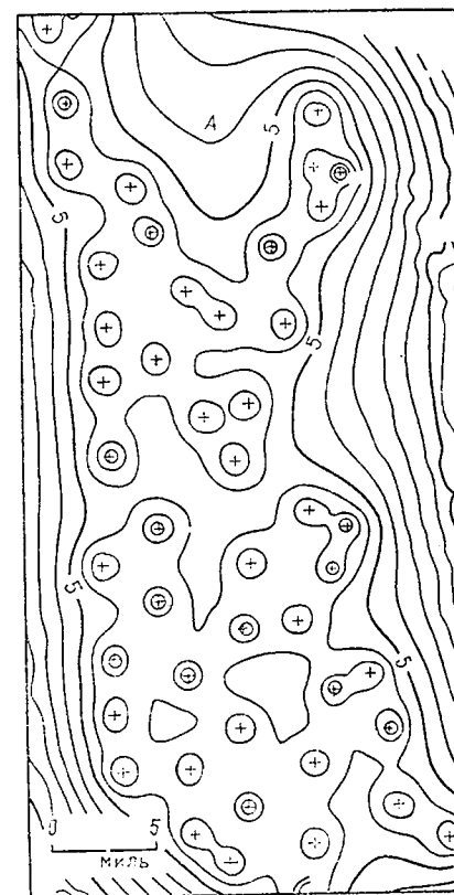
Рис. 5.68. На карте представлена стандартная ошибка оценок уровней воды в Экус Бедз.
