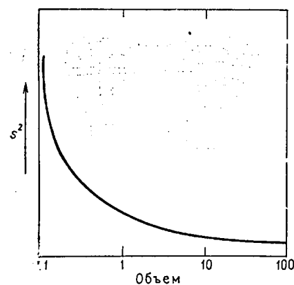
Рис. 5.61. Теоретическое изменение дисперсии содержаний полезного компонента в зависимости от изменений объема пробы или разрабатываемого блока
