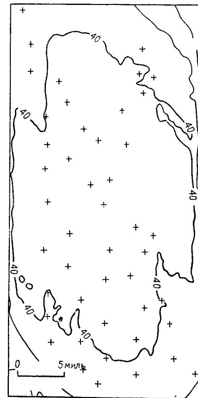
Рис. 5.70. Карта представляет стандартную ошибку дрифта первого порядка уровней воды в Экус Бедз.
