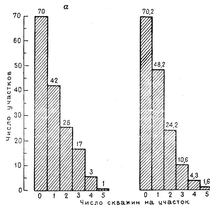
Рис. 5.13. Гистограммы, показывающие наблюдаемые числа разведочных скважин на участок на одной из площадей пермского бассейна (а) и ожидаемые числа в отрицательной биномиальной модели (б)
