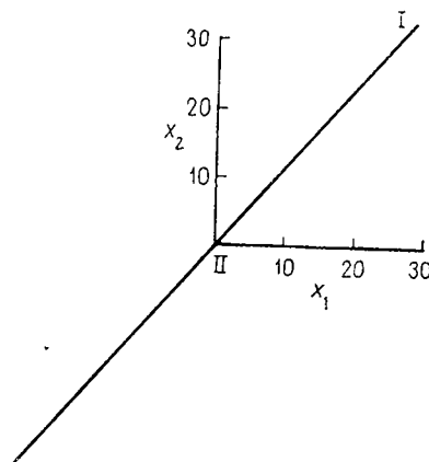
Рис. 6.24. Эллипс, определенный векторами дисперсий и ковариаций ранжированных данных рис. 6.23.
