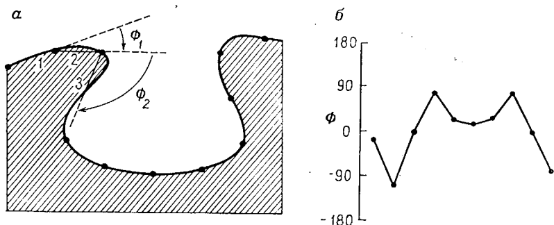
Рис. 5.42. Преобразование цифровых координат в угловые отклонения:
