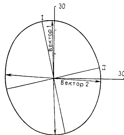
Рис. 6.26. Близкий к окружности эллипс, определенный векторами дисперсий и ковариаций для рандомизированных данных рис. 6.15.
