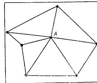
Рис. 5.46. Сеть треугольников Делоне вокруг точки А.
