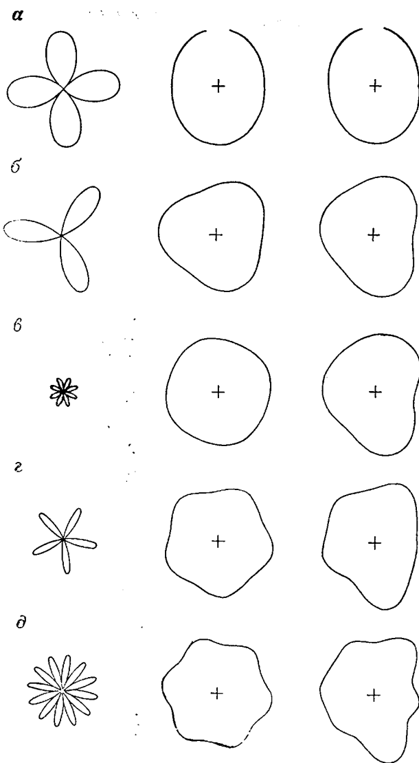
Рис. 5.38. Восстановление формы песчинки с помощью полярных рядов Фурье: a — вторая гармоника (слева), вторая гармоника плюс окружность, соответствующая среднему радиусу, или нулевая гармоника (центр), кумулятивная сумма гармоник (справа); б—г — соответственно третья, четвертая, пятая и шестая гармоники
