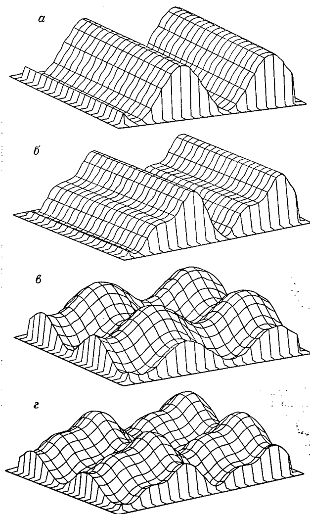
Рис. 5.91. Двумерные синусоидальные волны:
