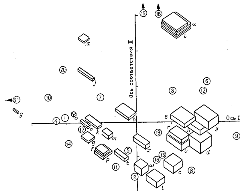
Рис. 6.47. Представление нагрузок R - и Q -методов на первые две оси соответствия для данных по блокам в порядке возрастания их объемов. Цифры в кружках — нагрузки R -метода (см. табл. 6.40. Значения 15, 18 и 21 — вне области диаграммы)
