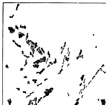
Рис. 5.82. Расположение основных нефтегазовых полей в центральном Канзасе
