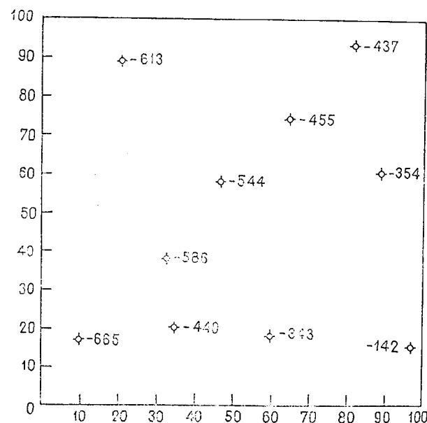
Рис. 5.73. Карта расположения скважин и абсолютных отметок подошвы меловых отложений в Северо-Восточной Африке. По данным нефтяной компании Англо-Баррен Ойл Кампани.
