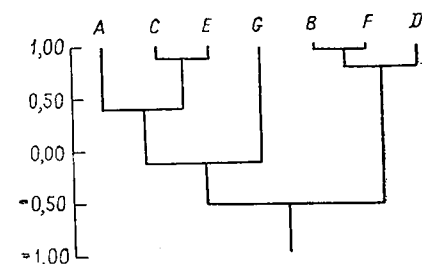
Рис. 6.11. Дендрограмма корреляционной матрицы, приведенной в табл. 6.15. Группы построены на основании невзвешенного усреднения. Коэффициент корреляции равен 0,72
