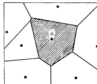
Рис. 5.45. Многоугольник Тиссена (заштрихован) вокруг точки А.
