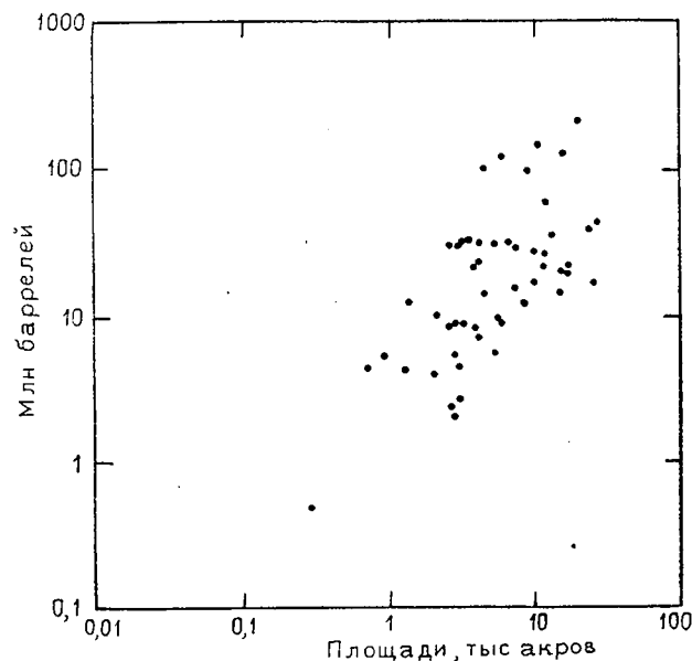
Рис. 2.39. Данные рис. 2.38, представленные в логарифмическом масштабе
