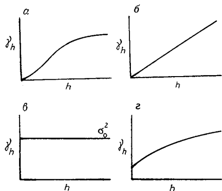
Рис. 4.45. Идеализированные полувариограммы:
