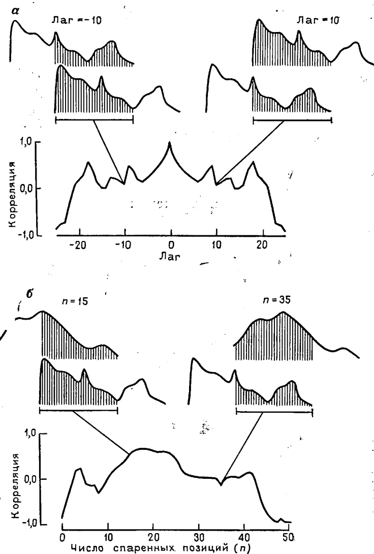
Рис. 4.34. Коррелограммы:
