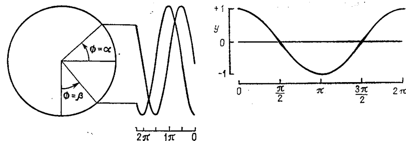
Рис. 4.52. Синусоидальная и косинусоидальная волны, соответствующие вращению диска.
