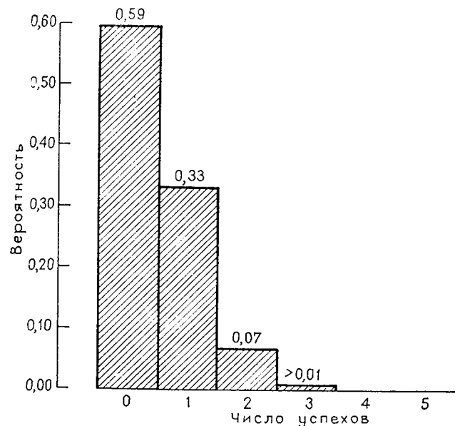
Рис. 2.3. Дискретное распределение, задающее вероятность успеха в программе бурения пяти скважин при условии, что вероятность успеха равна 10%
