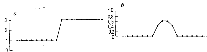
Рис. 4.61. Ступенчатая функция, состоящая из последовательностей единиц и троек (а). Графическое изображение первой производной ступенчатой функции, вычисленной на основе пятичленной квадратичной полиномиальной аппроксимации (б)
