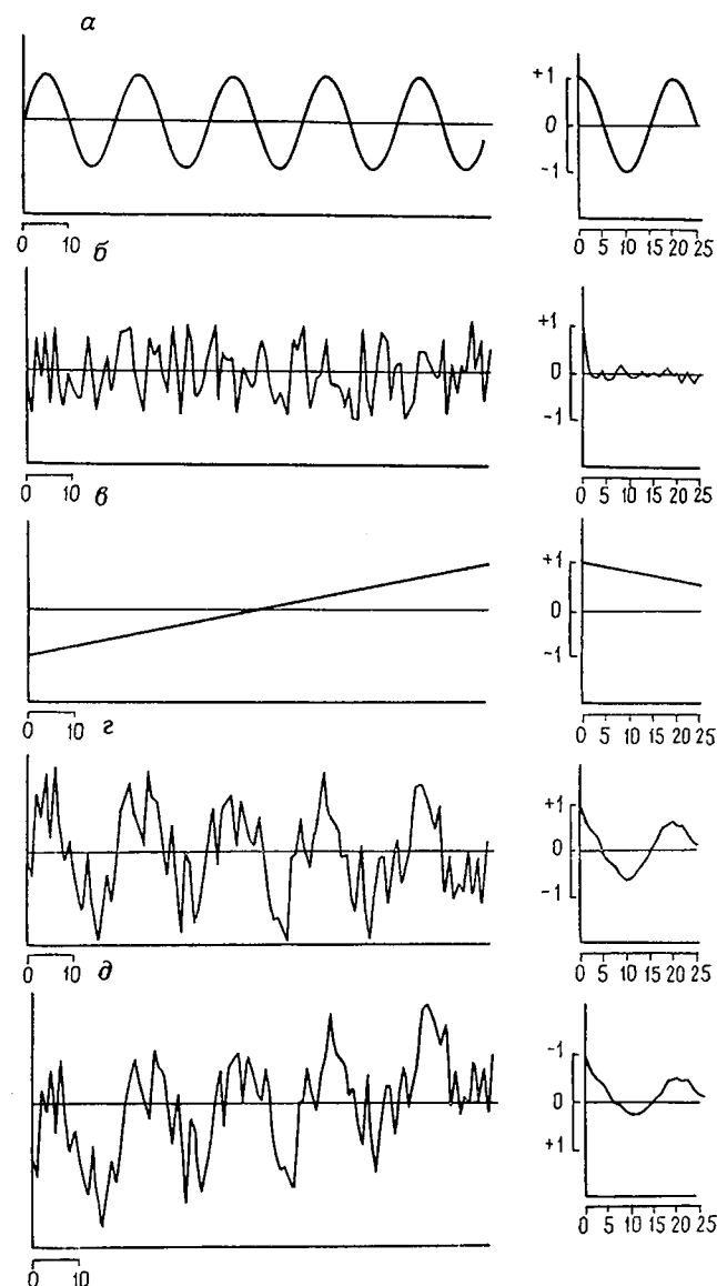
Рис. 4.33. Примеры идеализированных временных рядов и их автокорреляционные функции:
