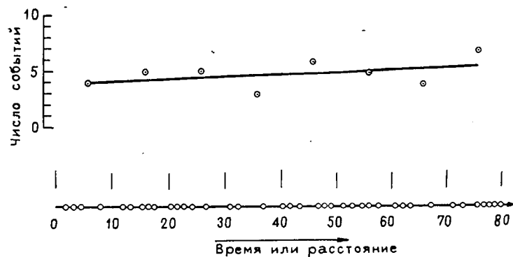
Рис. 4.10. Последовательности событий, которые происходят «мгновенно» в пространственном или временном континууме.
