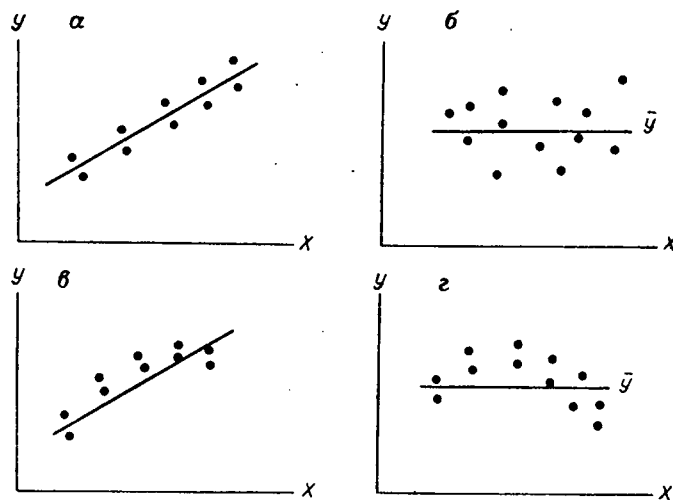
Рис. 4.17. Возможные случаи линейной регрессии [17]:
