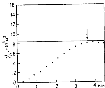
Рис. 4.41. Полувариограмма абсолютных отметок кровли меловой формации, измеренной вдоль морского сейсмического разреза в Магеллановом проливе, Чили [38].
