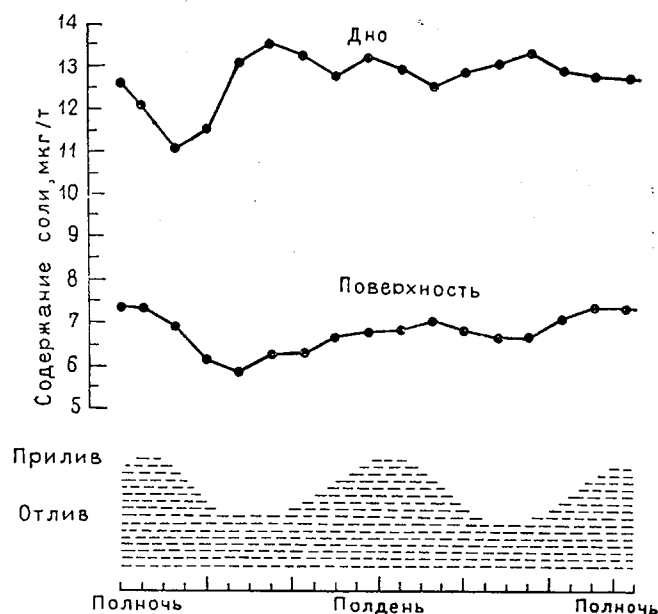
Рис. 4.38. Содержания соли в придонных водах и поверхностных водах и Шизапик Бей вблизи Аннаполиса (штат Мэриленд)
