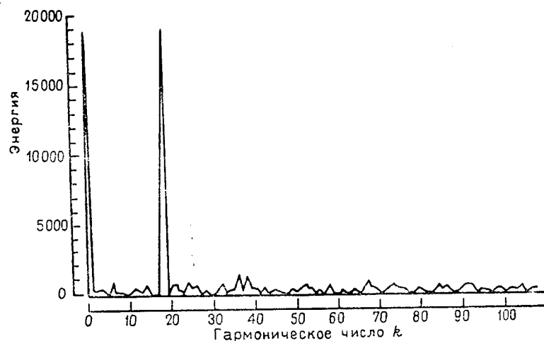
Рис. 4.55. Периодограмма месячного потока Кейв-Крик, Кентукки.
