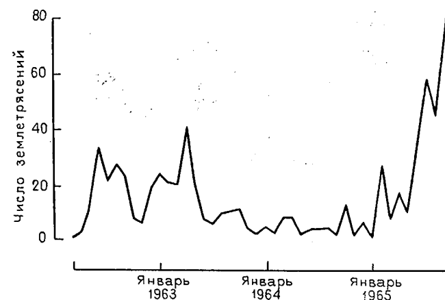
Рис. 4.36. Число зарегистрированных в течение месяца землетрясений, эпицентр которых был расположен вблизи Денвера (штат Колорадо)
