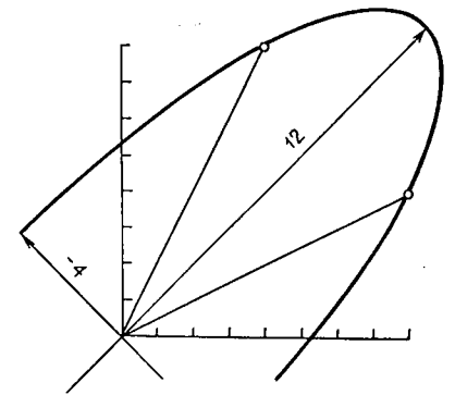
Рис. 3.2. Эллипс, определенный элементами матрицы порядка 2 \times 2 . Собственные векторы матрицы соответствуют главным полуосям эллипса
