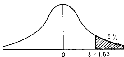
Рис. 2.30. Распределение Стьюдента с девятью степенями свободы
