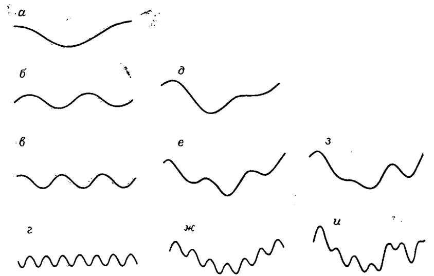
Рис. 4.54. Результат сложения последовательных гармоник косинусоидальной волны.
