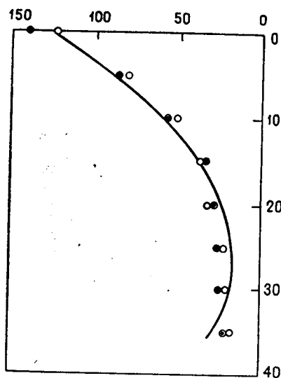
Рис. 4.20. Кривая полиномиальной регрессии второй степени, полученная по замерам влажности, взятым из таблиц 4.11 и 4.14
