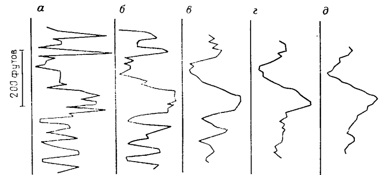
Рис. 4.60. Результаты сглаживания последовательности значений каротажной диаграммы в скважине с помощью различных уравнений [26, рис. 4.2]: а — исходные данные; б—д — число членов: 5 (б), 9 (в), 13 (г), 17 (д)
