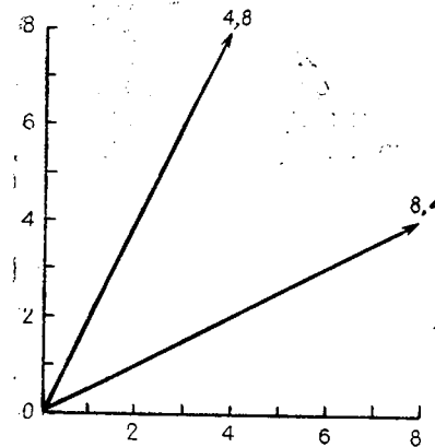
Рис. 3.1. Два вектора, определенные элементами порядка матрицы 2 \times 2
