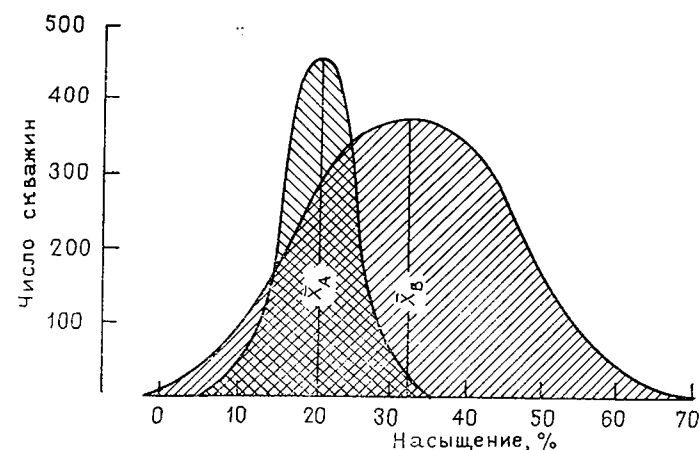
Рис. 2.11. Частотное распределение процентного содержания насыщения нефтью в нефтяном поле Оклахомы (A) и Техаса (B)
