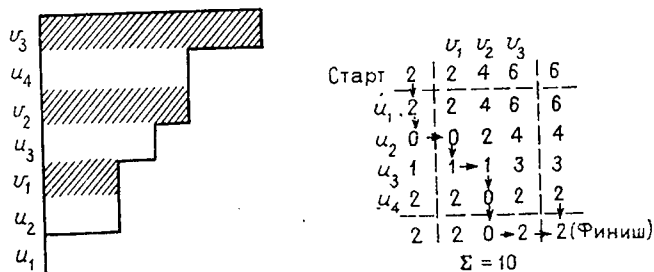
Рис. 4.29. Оптимальное объединение последовательностей U и V .
