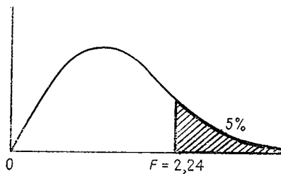
Рис. 2.31. Типичное F -распределение с v_1=10 и v_2=25 степенями свободы и заштрихованной критической областью, составляющей 5% площади под кривой
