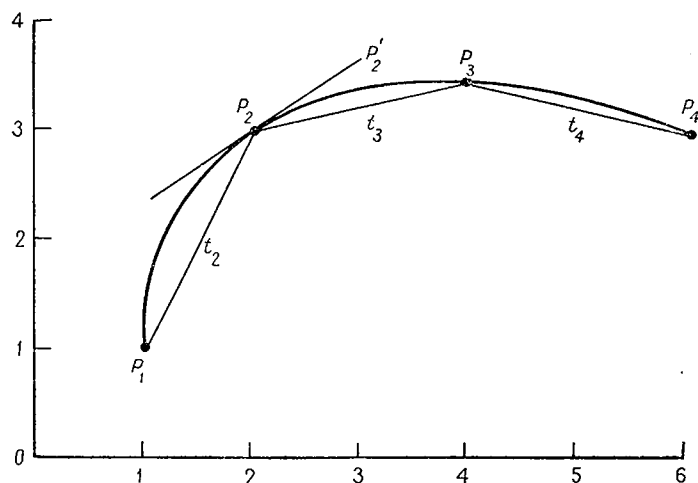
Рис. 4.23. Четыре точки, связанные функцией кубического сплайна. Исходные наблюдения обозначены через P_i . Расстояния по хордам между точками равны t_i . Касательная к сплайну во внутренней точке P_2 обозначена через P_2' .
