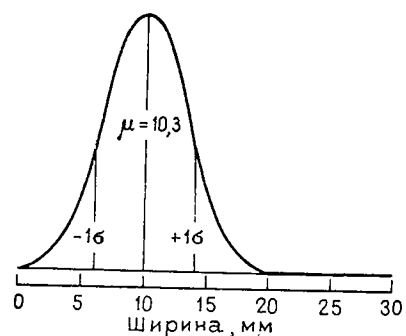
Рис. 2.20. Гипотетическое распределение значений ширины особей рода Composita
