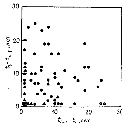
Рис. 4.9. Сериальная корреляция продолжительностей между последовательными изображениями вулкана Асо.
