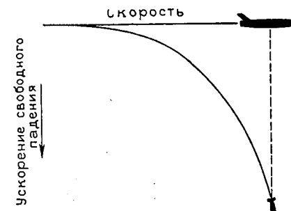
Рис. 4.18. Теоретическая траектория падения бомбы, сброшенной с самолета
