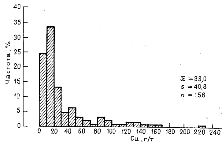
Рис. 2.35. Гистограмма содержания меди в осадочных породах на площади Нансен в Юконе [29]
