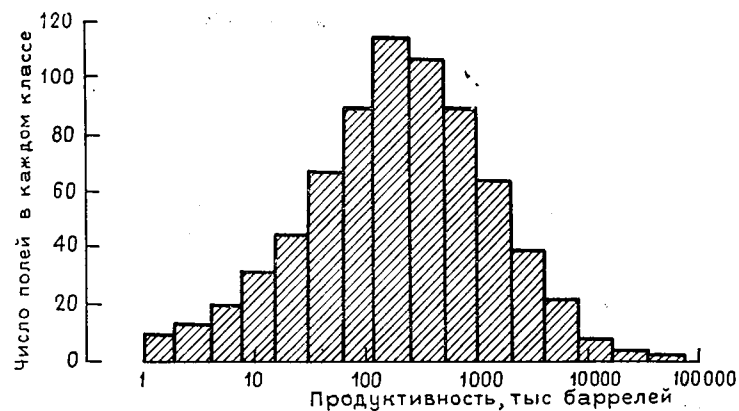
Рис. 2.36. Гистограмма распределения продуктивности нефтеносных полей, открытых в Денверском бассейне в 1969 г. Масштаб логарифмический. Взято из Харбуха, Давтока, Девиса
