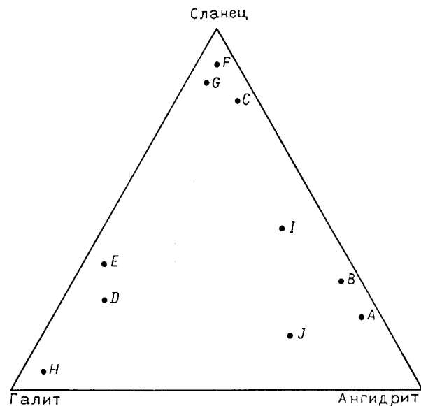
Рис. 2.18. Треугольная диаграмма галит—ангидрит—сланец как композиционная система. Точки характеризуют средние содержания пород Веллингтонской формации (пермь), извлеченных из скважин в Центральном Канзасе с интервалом 1,5 м
