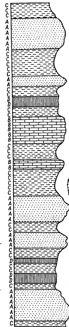
Рис. 4.4. Стратиграфический разрез, в котором литологические состояния взаимно исключают друг друга: A — песчаник; B — известняк; C — сланец; D — уголь
