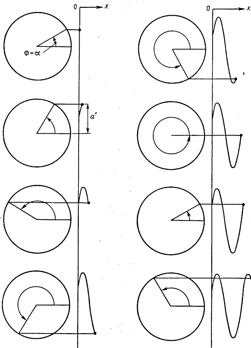
Рис. 4.51. Постепенное изменение фазового угла от начального значения \Phi . Для последовательных значений x_i , Y_i = A \sin(2\pi x_i / X + \Phi) и \alpha_i = 2\pi x_i / X + \Phi
