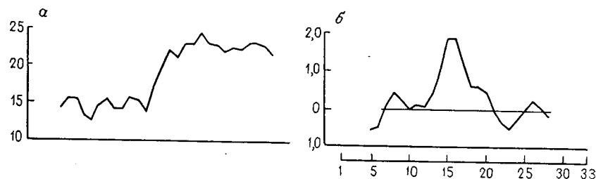
Рис. 4.63. Сглаженные значения пористости из арктической скважины: а — данные, сглаженные с помощью пятичленного квадратичного многочлена; б — первая производная сглаженных данных
