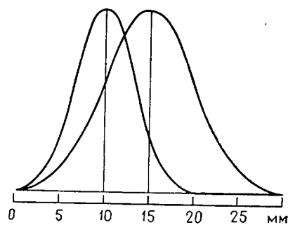
Рис. 2.21. Диаграмма распределения значений длины и ширины особей рода Composita
