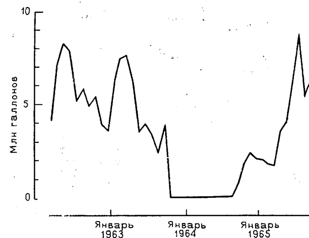
Рис. 4.35. Количество отравленной жидкости, закачанной в скважину в Скалистых горах
