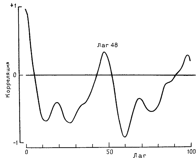
Рис. 4.32. Автокоррелограмма гамма-каротажа, изображенного на рис. 4.30
