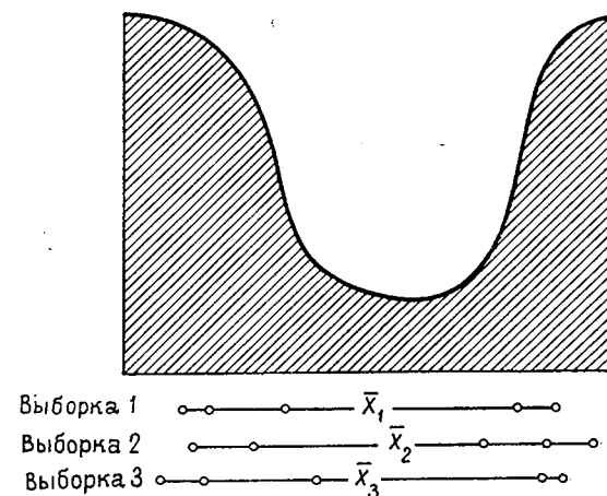
Рис. 2.24. Три выборки из пяти наблюдений, взятые наудачу из совокупности с U-образным распределением. Средние значения выборок обозначены через \bar{X}
