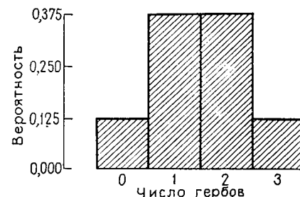
Рис. 2.2. Дискретное распределение, показывающее вероятность получения заданного числа гербов при трех бросаниях монеты
