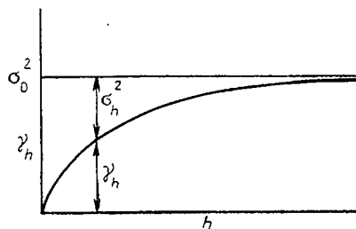
Рис. 4.43. Соотношение между полудисперсией \gamma_h и автоковариацией для стационарной регионализованной переменной.
