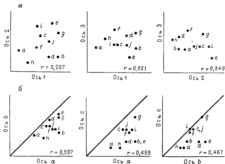
Рис. 2.17. Диаграмма рассеяния длин осей (в см) образцов гальки, отобранных на галечном пляже:
