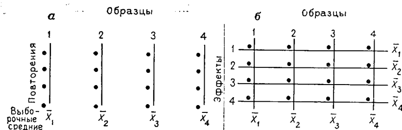
Рис. 2.32. Схемы суммирования в дисперсионном анализе: а — однофакторный дисперсионный анализ; суммирование для нахождения выборочного среднего производится сверху вниз по столбцам; б — двухфакторный дисперсионный анализ; суммирование для нахождения выборочных средних производится как по строкам, так и по столбцам
