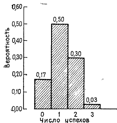
Рис. 2.6. Дискретное распределение, задающее вероятность p успехов в трех скважинах из десяти, если четыре из десяти пересекали нефтяную залежь
