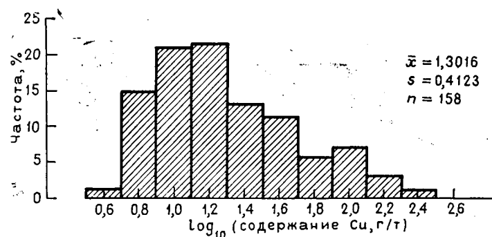
Рис. 2.37. Гистограмма содержаний меди в осадочных породах на площади Нанси в Юконе. Представлена в логарифмическом масштабе [29]
