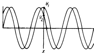
Рис. 4.49. Две синусоидальные волны, которые идентичны по форме.
