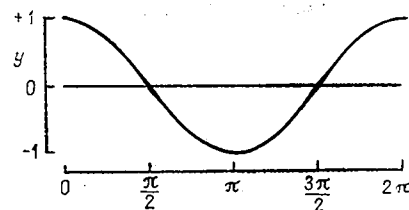
Рис. 4.53. Синусоидальная волна. Общая длина кривой равна 2\pi радиан
