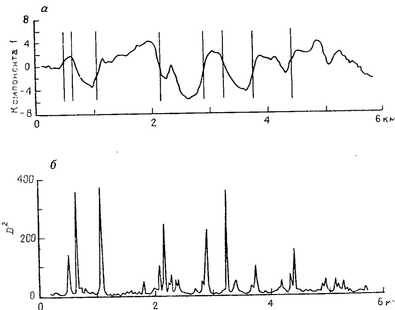
Рис. 4.26. Сечение, на котором указаны изменения свойств почвы вдоль 6-километровой линии в верхней части Теймс Вэлли (Англия): а — изменение 27 свойств по первой главной компоненте; б — значение D^2 вдоль траверса. Максимумы определенных границ указаны на графике а
