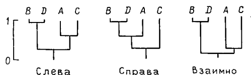
Рис. 4.65. Группы стратиграфических состояний, построенные по трем типам мер взаимозаменяемости.
